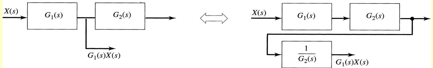
(d) Moving a pickoff point forward
