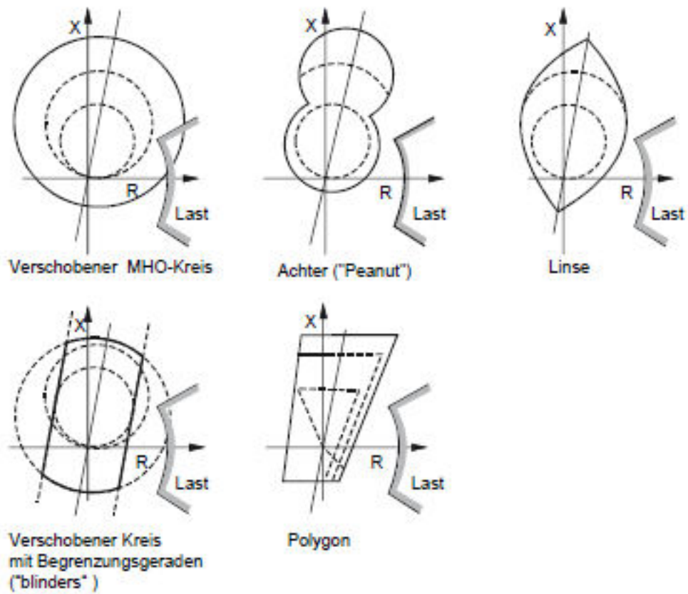
Bild 3.18 Impedanzanregung in konventioneller Technik
